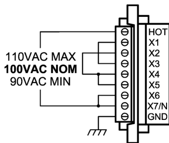
100VAC HOOKUP
