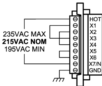
215VAC HOOKUP
